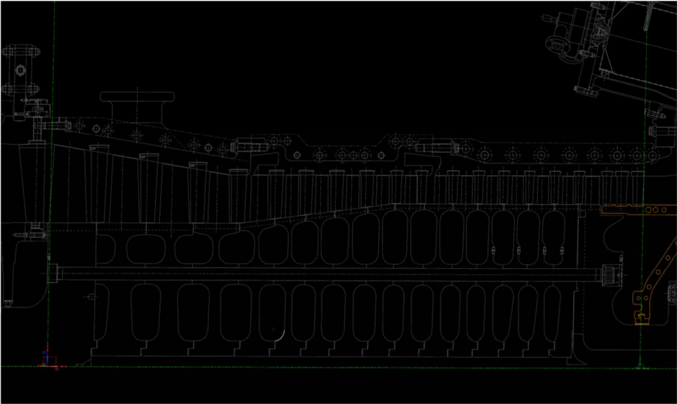
9E Cross Section
